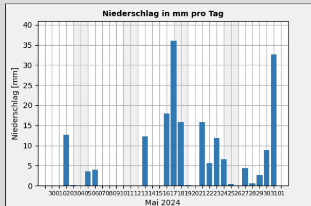
Gr. 3: Niederschlagssumme in mm pro Tag vom 01.05. - 31.05.2024; Quelle: Wetterstation der Sternwarte "Welzheim"*
