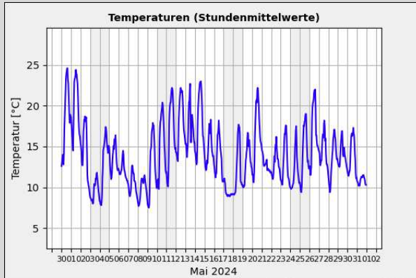
Gr. 1: Temperaturmittelwerte pro Std. in °C vom 01.05. - 31.05.2024; Quelle: Wetterstation der Sternwarte "Welzheim"*
