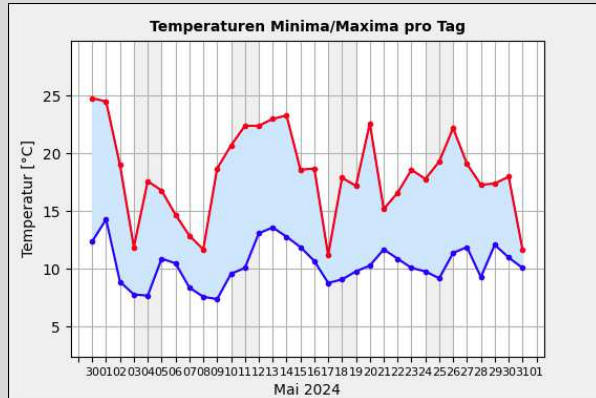
Gr. 2: Temperaturhöchst- u. -tiefstwerte pro Tag in °C vom 01.05. - 31.05.2024; Quelle: Wetterstation der Sternwarte "Welzheim"*
